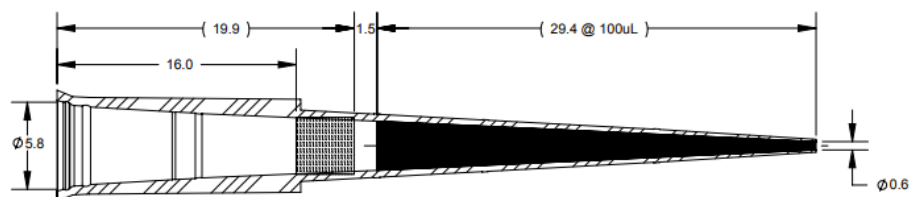
SECTION A-A SCALE: 3 : 1
